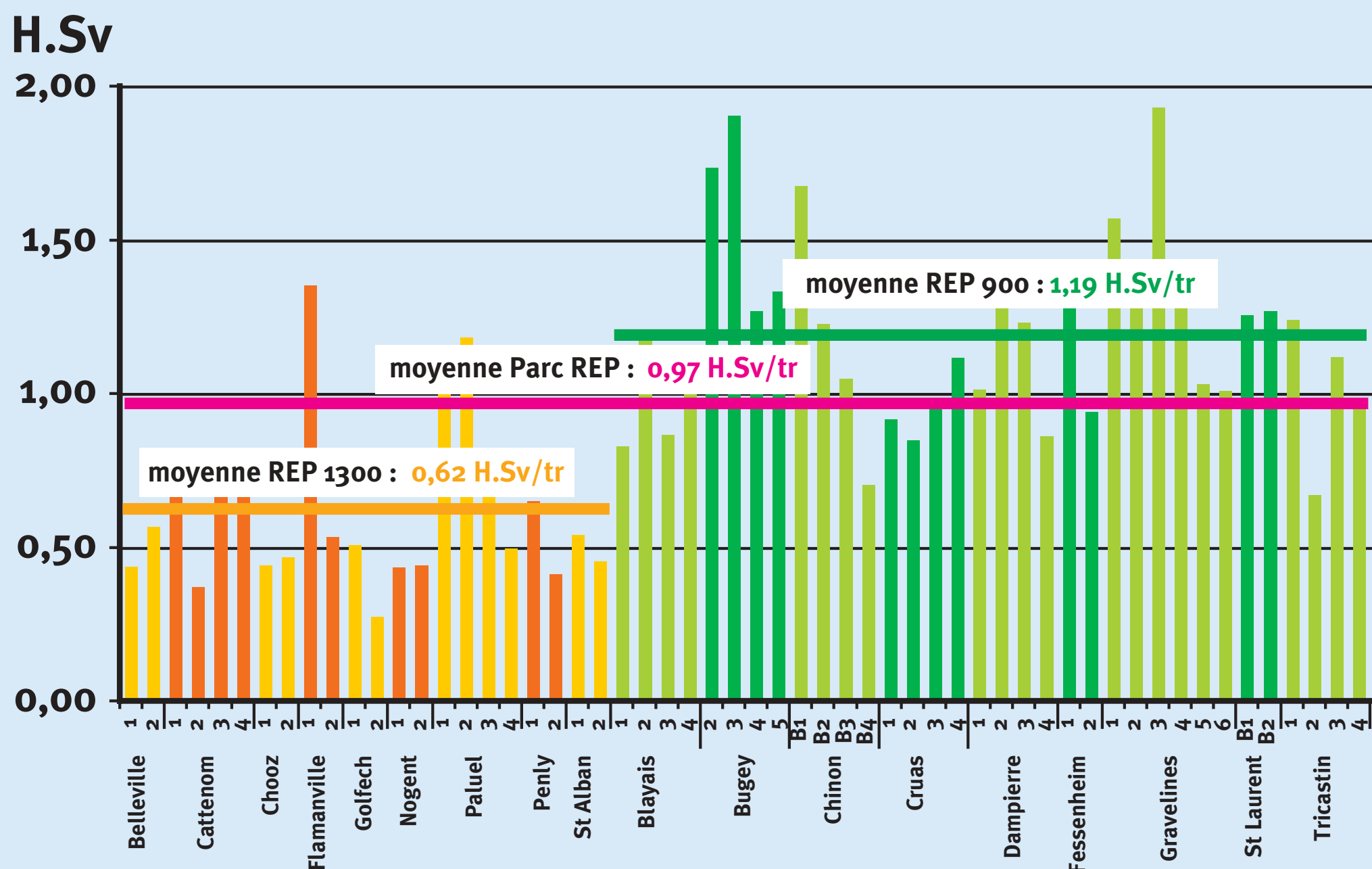
Dose collective par réacteur du Parc REP moyenne sur 3 ans (2001, 2002 et 2003)
