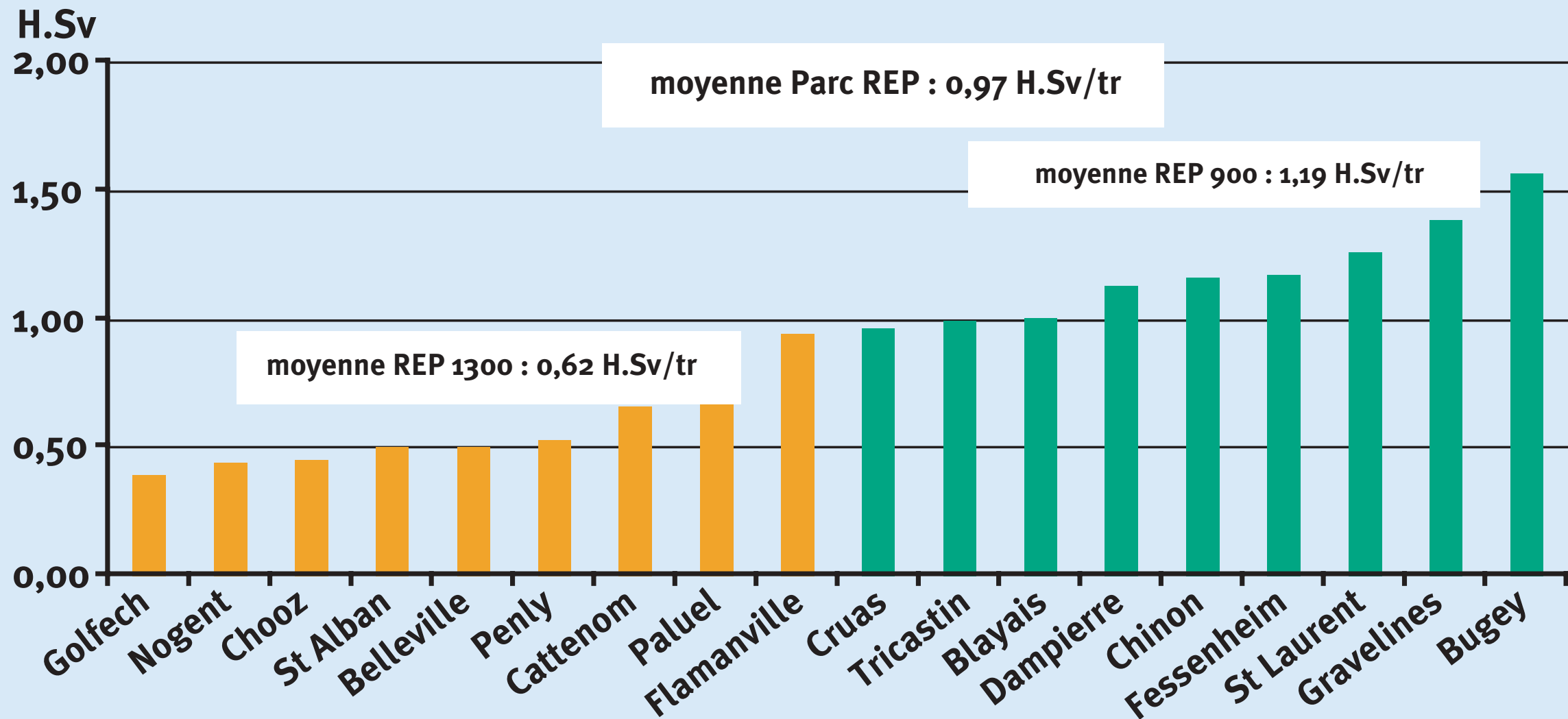
Dose collective par site ramenée par réacteur moyenne sur 3 ans (2001, 2002 et 2003)
